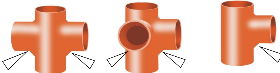
Exemple de raccords avec angle d'écoulement de 45° Formstücke 88° mit Einlaufwinkel 45°
